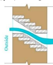
شکل ۱. مقطع از اندام اقلیمی سورک (Heidari et al., 2017)
