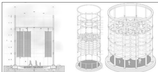
ت ۲۰. جزئیات طراحی برج دیدبانی چارک با قابلیت استحصال آب از مه (ytaa.miesbcn.com, 2020)
