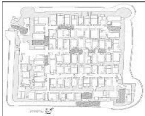
ت ۴. پلان قلعه خویدک (آرشیو اداره کل میراث فرهنگی، صنایع دستی و گردشگری استان یزد: ۱۳۸۳).
