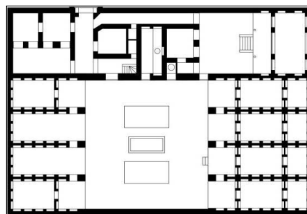
ت ۱. نمای آفتاب‌روی و پلان خانه کارشناس از گونه دهانه‌ای
