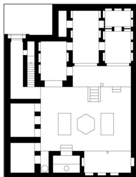
ت ۲. نمای ایوان و پلان خانه کبیرزاده از گونه کشابی
