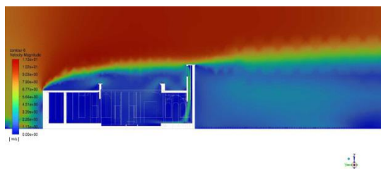
شکل ۱۶. مقطع ساختمان و نحوه ورود هوا به فضای مورد بررسی، حالت وضع موجود
