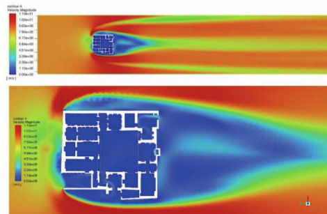
شکل ۱۵. پلان نحوه توزیع باد در فضای مورد بررسی، حالت وضع موجود
