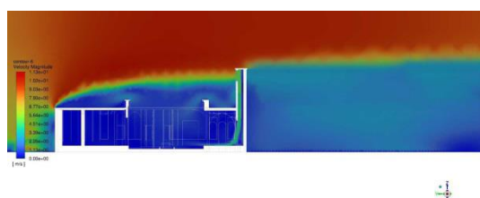
شکل ۱۸. مقطع نحوه توزیع باد در فضای مورد بررسی، حالت بادگیر با ارتفاع بیشتر
