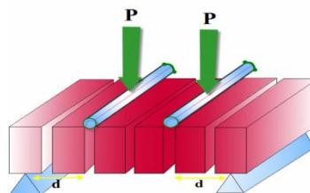
ت ۹. شمای آزمایش خمشی بر روی نمونه‌های منشوری ساخته شده با ۶ ردیف خشت.
