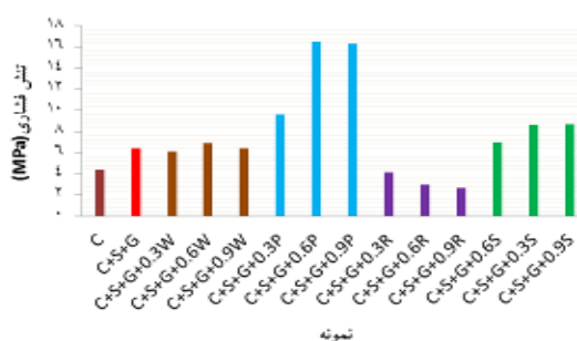
ن ۵. نمودار مقایسه نتایج نمونه‌های با افزودنی طبیعی.
