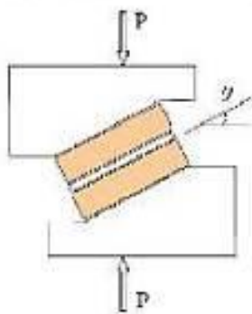
ت ۱۰. شمای آزمایش مقاومت برشی مصالح بنایی.
