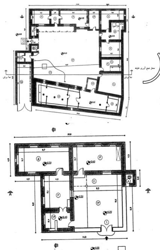
نقشه شماره ۲: نمونه پلانهای U و L شکل در گونه دشتی؛ ماخذ: مطالعات جهاد دانشگاهی تهران
