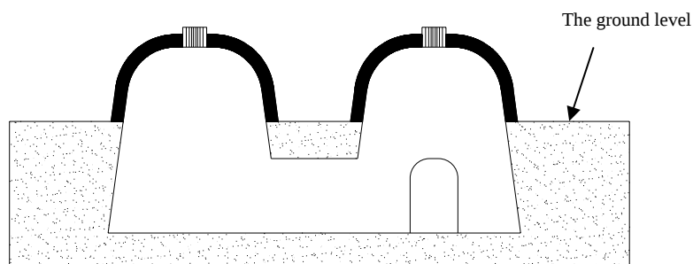
تصویر شماره ۸: عنصر فضایی-عملکردی زاغه در گونه دشتی (روستاهاى قلعه کهنه و احمدآباد دیواندره)
