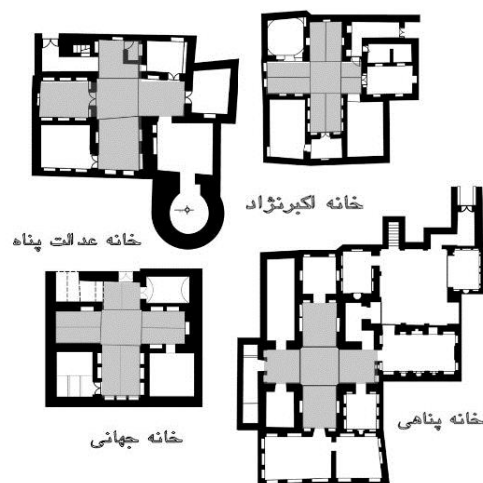
ت ۱۰. تهرانگ برخی از خانه‌های چهارصفه. مأخذ: پایگاه میراث فرهنگی شهر تاریخی بشرویه.
