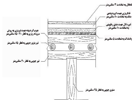
جزئیات اجرایی اتصال ستون چوبی به تیر چوبی
