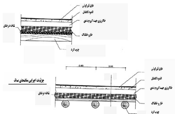
"ت ۷" جزئیات اجرایی سقف‌های تیر پوش چوبی .
