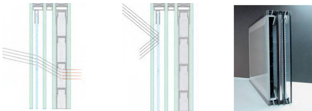
تصویر ۲۱: مقطع از پنجره با عایق هیدرات نمک، تابستان و زمستان (Ritter, 2007)
