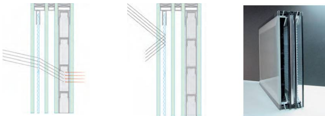
تصویر ۲۱: مقطع از پنجره با عایق هیدرات نمک، تابستان و زمستان (Ritter, 2007)
