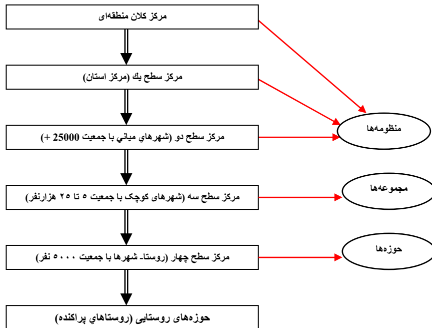
نمودار شماره ۲: الگوی پیشنهادی نظام سلسله مراتب سکونتگاهی
