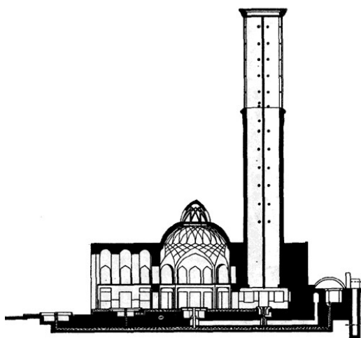
تصویر شماره ۸: مقطع از بادگیر یکی از خانه‌های یزد مأخذ: www.picestoon.com
