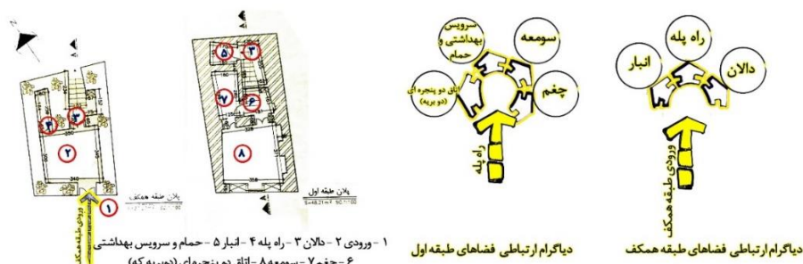
شکل ۱۲. تحلیل فضایی خانه‌های گسترش یافته در ارتفاع پنجره دار با یک اتاق در عرض ماسوله
