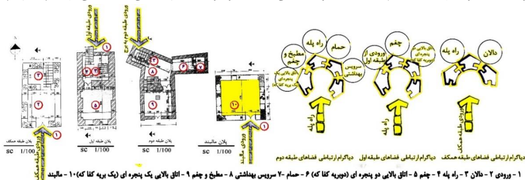
شکل ۹. تحلیل فضایی و جانمایی مال بند در بنای مسکونی ماسوله
