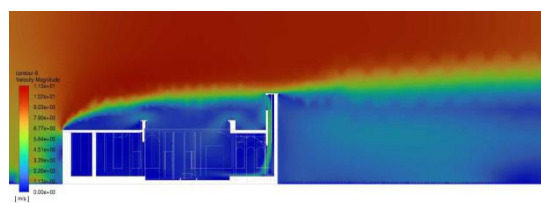
شکل ۱۶. مقطع ساختمان و نحوه ورود هوا به فضای مورد بررسی، حالت وضع موجود
