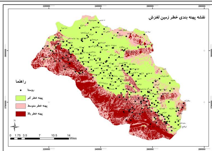
شکل ۴. نقشه پهنه‌بندی خطر زمین لغزش
