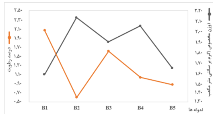
شکل ۳. مقایسه روند تغییرات میزان رطوبت و وزن مخصوص نمونه‌های آجری به ترتیب دوره زمانی
