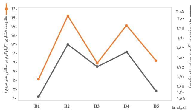
شکل ۷. مقایسه دو نمودار مقاومت فشاری و وزن مخصوص نمونه‌های آجری به ترتیب دوره زمانی
