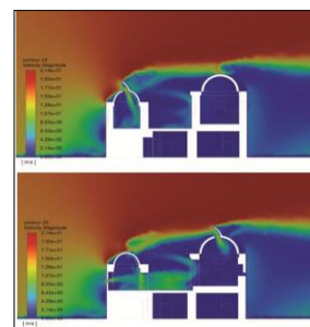
ت ۲۰. مقطع ساختمان و نحوه ورود هوا به اتاق‌ها - حالت باد عمود بر دهانه کُلک
