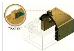
ت ۲. طرح‌واره اندام کُکک و جانمایی آن‌ها در کالبد یک مسکن روستایی. منبع: Heidari et al., 2017
