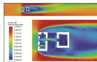
ت ۱۹. تصویر نحوه توزیع باد در اتاق‌های مورد بررسی - حالت باد عمود بر دهانه کُلک
