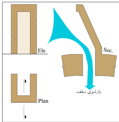
ت ۳. نحوه عملکرد کُکک در تهویه طبیعی (تصویر سمت راست: مقطع و تصویر سمت چپ بالا: نما و چپ پایین: پلان)
