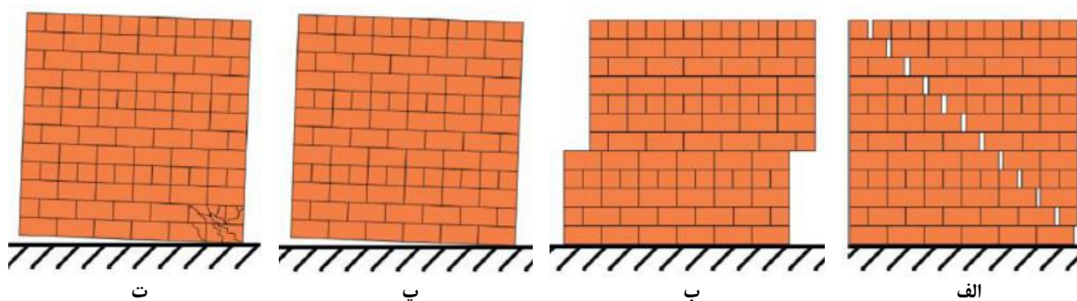
شکل ۲. مدهای گسیختگی مختلف دیوارهای مصالح بنایی. الف. برشی؛ ب. برشی-لغزشی؛ پ. گهواره‌ای یا خمشی؛ ت. خردشدگی پاشنه
