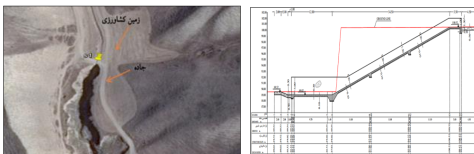
ت ۴. نمایی از موقعیت سازه‌های مکانیکی آبخیزداری طراحی شده به همراه برخی جزئیات سازه‌ای
