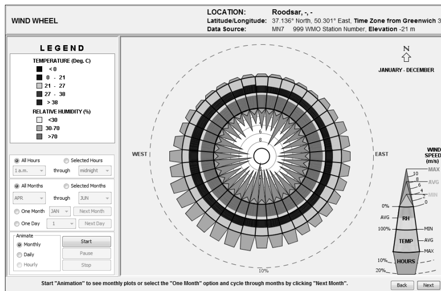
ت ۴. متوسط سالانه گلباد شهر رودسر (براساس نرم افزار کلایمت کانسلانت)
