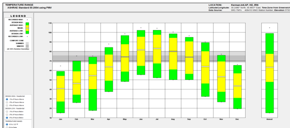
ت۲. نمودار نوسان دمای خشک در شهر کرمان در مقایسه با شرایط آسایش حرارتی در استاندارد اشری ۸ ، استخراج شده از نرم افزار مشاور اقلیمی ۹
