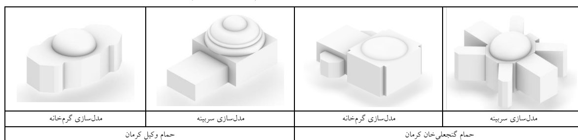
ج ۲. مدل‌سازی پوسته داخلی فضاهای سرپینه و گرم‌خانه در حمام‌های منتخب پژوهش
