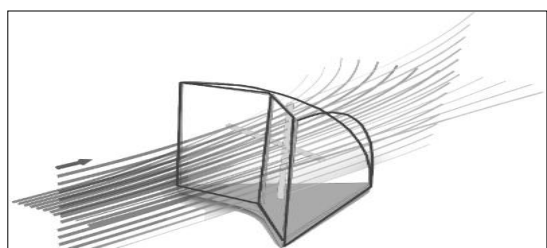
ت ۲۷. شبیه‌سازی تونل باد غالب روستای امین‌آباد در زمان برخورد با دستگاه و تغییر جریان هوا از داخل آن را نشان می‌دهد
