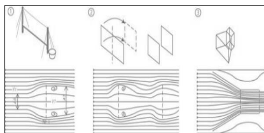
ت۱۷. فرایند مدل طراحی سیستم برداشت مه: ۱) دستگاه برداشت مه سستی که در آن جریان باد قابل‌توجهی توسط مش مسطح منحرف می‌شود. ۲) مش دو لایه پیشنهادی که در آن جمع‌آوری با افزایش جریان باد افزایش می‌یابد. ۳) ساختار قیفی که باد را تماماً در خود می‌کشد و امکان جمع‌آوری آب بسیار بیشتری را فراهم می‌کند (Fernandez et al., 2019, 542)
