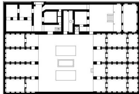
ت ۱. نمای آفتاب‌روی و پلان خانه کارشناس از گونه دهانه‌ای
