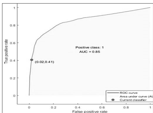
ت۱۵. روش Medium tree
