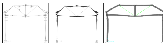
ت ۲۲. تغییر شکل سازه تحت اثر بارهای ثقلی. ت ۲۳. ممان خمشی سازه.
