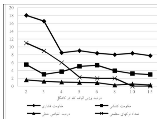
ن ۵. نتایج آزمایش نمونه‌های کاهگل با درصد‌های مختلف الیاف کاه.
