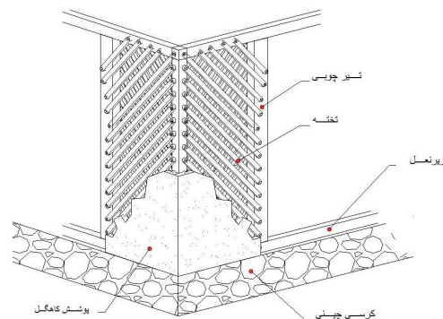
ت 13. جزئیات اجرای خانه‌های لارده‌ای. منبع: نگارندگان.
