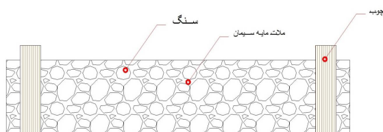
ت 8. نحوه اجرای کرسی چینی. منبع: نگارندگان.
