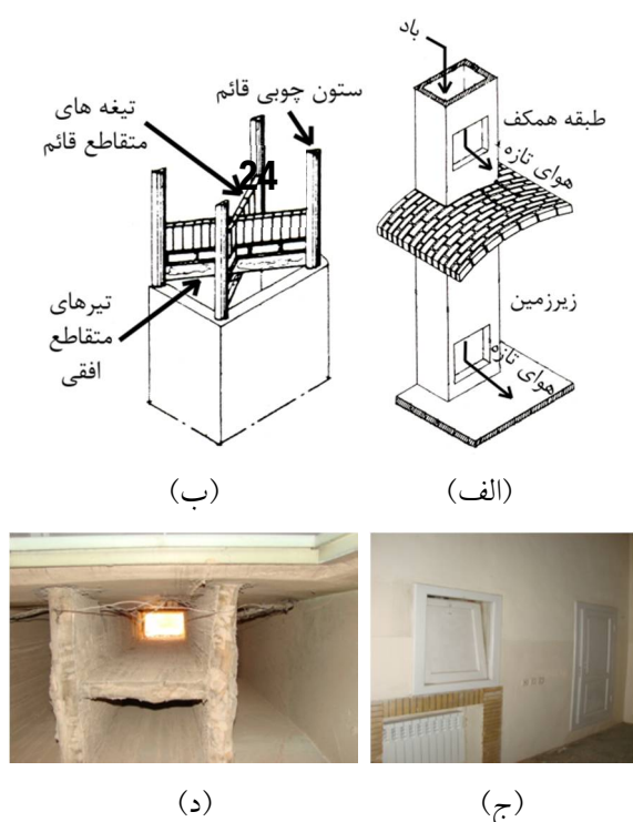
ت 1. روش ساخت بادگیر: الف) کانال (زمرشیدی، 1381)، ب) عناصر سازه‌ای (زمرشیدی، 1381)، ج) بازشو در اتاق نشیمن، د) تیغه‌های قائم داخل کانال.
