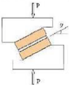
ت ۱۰. شمای آزمایش مقاومت برشی مصالح بنایی.
