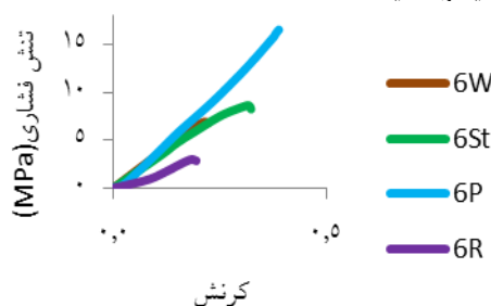
ن ۳. نمودار مقایسه نتایج نمونه‌های با ۰/۶ درصد افزودنی طبیعی.
