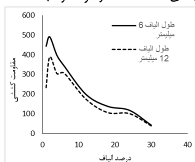
شکل ۵. مقایسه مقاومت کششی نمونه‌های خشتی با درصد الیاف مختلف در دو طول لیف ۶ و ۱۲ میلی‌متر
