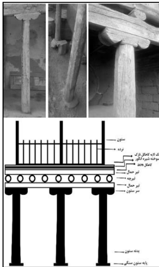
ت ۱۶. جزئیات اجرای ساختار ستون در خانه‌های تاریخی و سنتی روستای سپورغان (مأخذ: نگارندگان).
