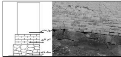
ت ۱۴. جزئیات اجرایی کرسی چینی و دیوار در خانه‌های تاریخی و سنتی روستای سپورغان (مأخذ: نگارندگان).
