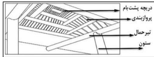
ت ۱۵. نمونه سقف واحدهای همکف خانه‌های تاریخی و سنتی روستای سپورغان (مأخذ: نگارندگان).
